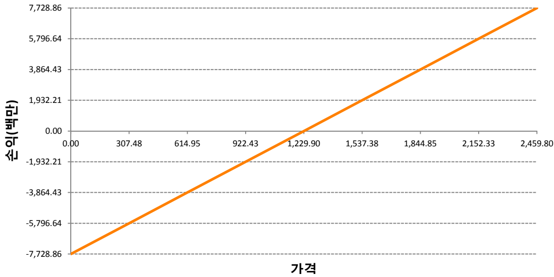
LBMA20200420-LBMA골드ICBC20200420
