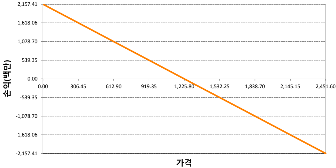
KR4175Q40008-2020-04 달러선물
